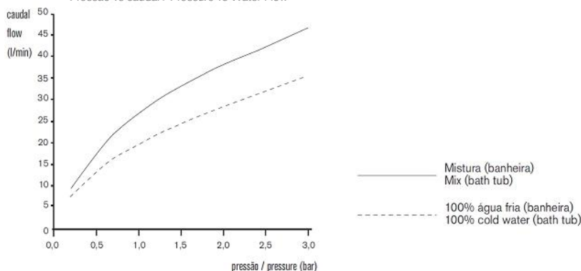
Pressão vs caudal / Pressure vs Water Flow
